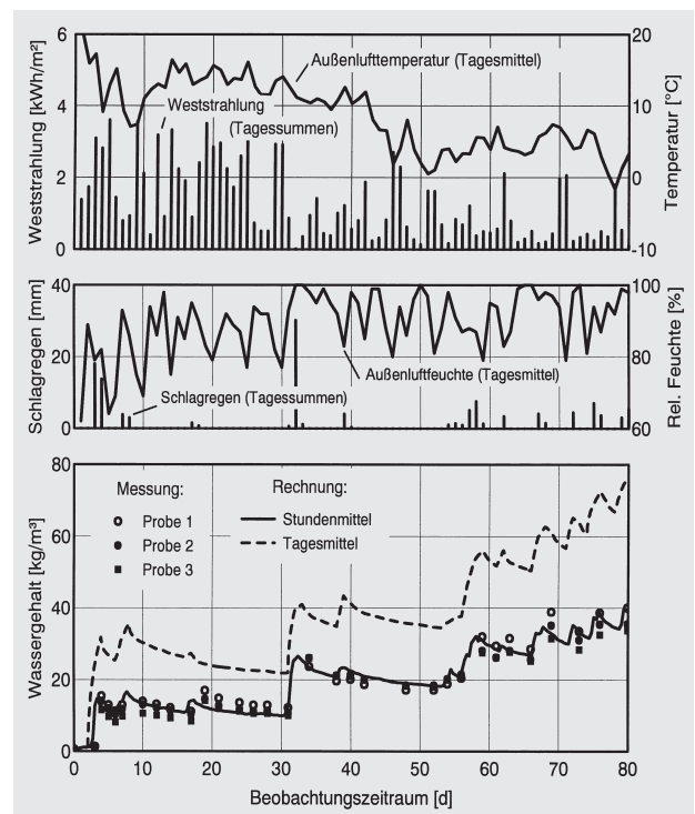
Bild 1: Berechneter Zeitverlauf des Wassergehalts einer 25 cm dicken Westwand aus Natursteinmauerwerk im Vergleich zu Messungen an 3 Natursteinfassadenproben mit Angabe der im Beobachtungszeitraum vorhandenen meteorologischen Randbedingungen. Oben: Gemessener Verlauf der Strahlungsintensität und der Außenlufttemperatur. Mitte: Gemessener Verlauf des Schlagregens und der relativen Feuchte der Außenluft. Unten: Wassergehaltsverlauf (berechnet und gemessen).
