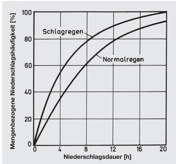
Bild 2: Summenhäufigkeit der im Zeitraum von fünf Jahren aufgetretenen Schlagregen- und Normalregenmengen in Holzkirchen, aufgetragen über der Dauer der Niederschlagsereignisse. Der Schlagregen wurde durch einen in die Westfassade einer etwa 4 m hohen Versuchshalle integrierten, kontinuierlich arbeiteten Tropfenzähler in 1,5 m Höhe bestimmt.
